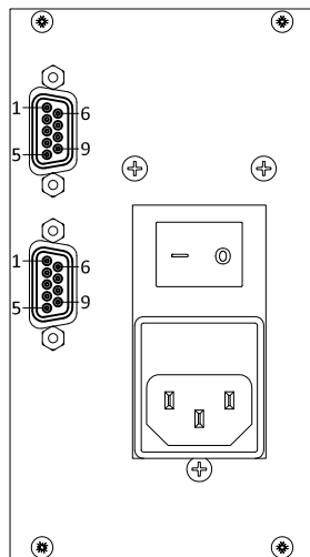
Connecteur D-sub 9 broches femelle (2x)
